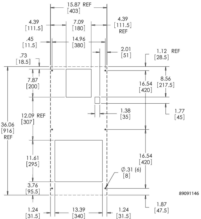
CUTOUT DIMENSIONS
